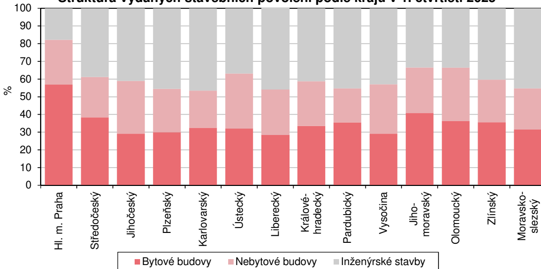
Struktura vydaných stavebních povolení podle krajů v 1. čtvrtletí 2025
